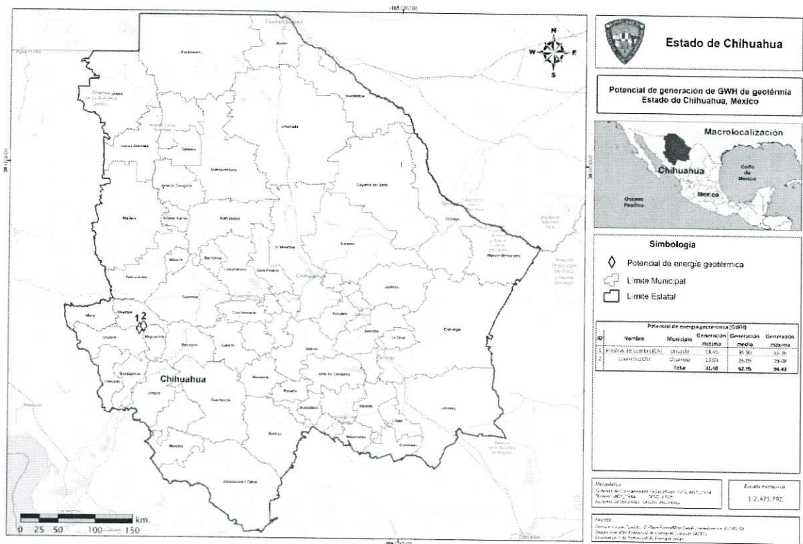
Mapa 3. Municipios del estado de Chihuahua con potencial de Energía Geotérmica
