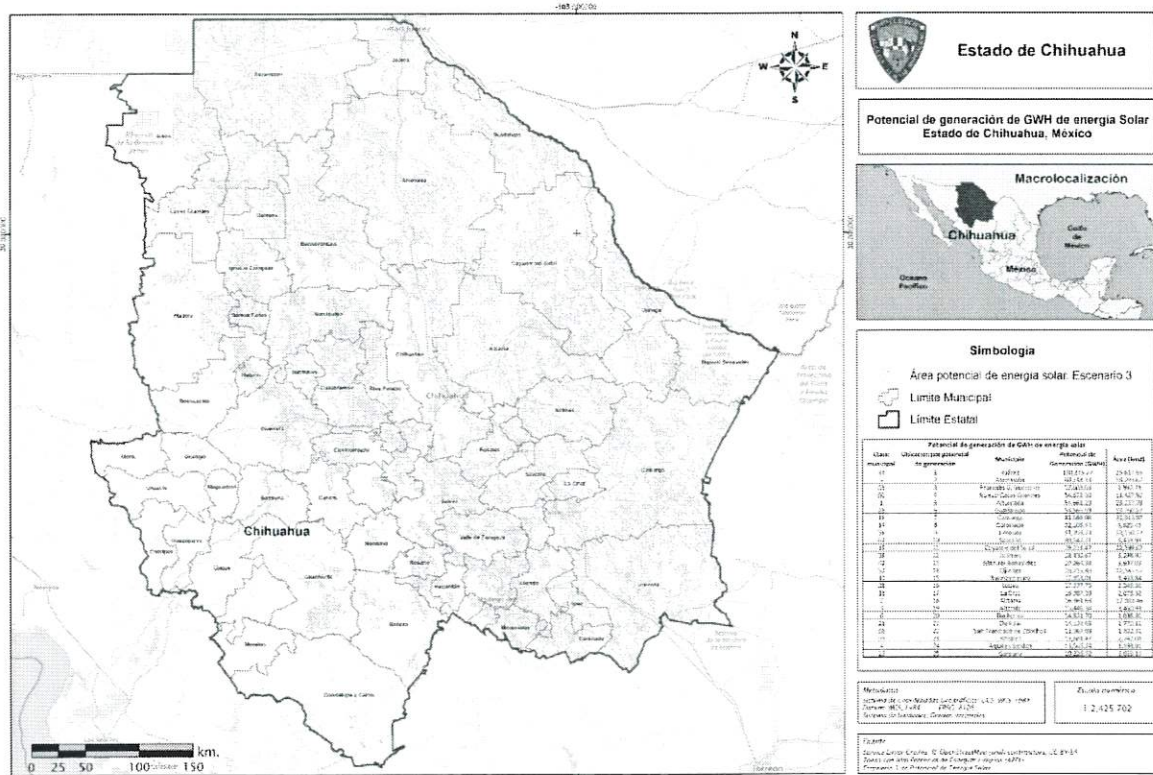
Mapa 2. Municipios del estado de Chihuahua con potencial de Energía Solar
