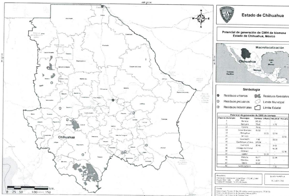
Mapa 2. Municipios del estado de Chihuahua con potencial de biomasa.
